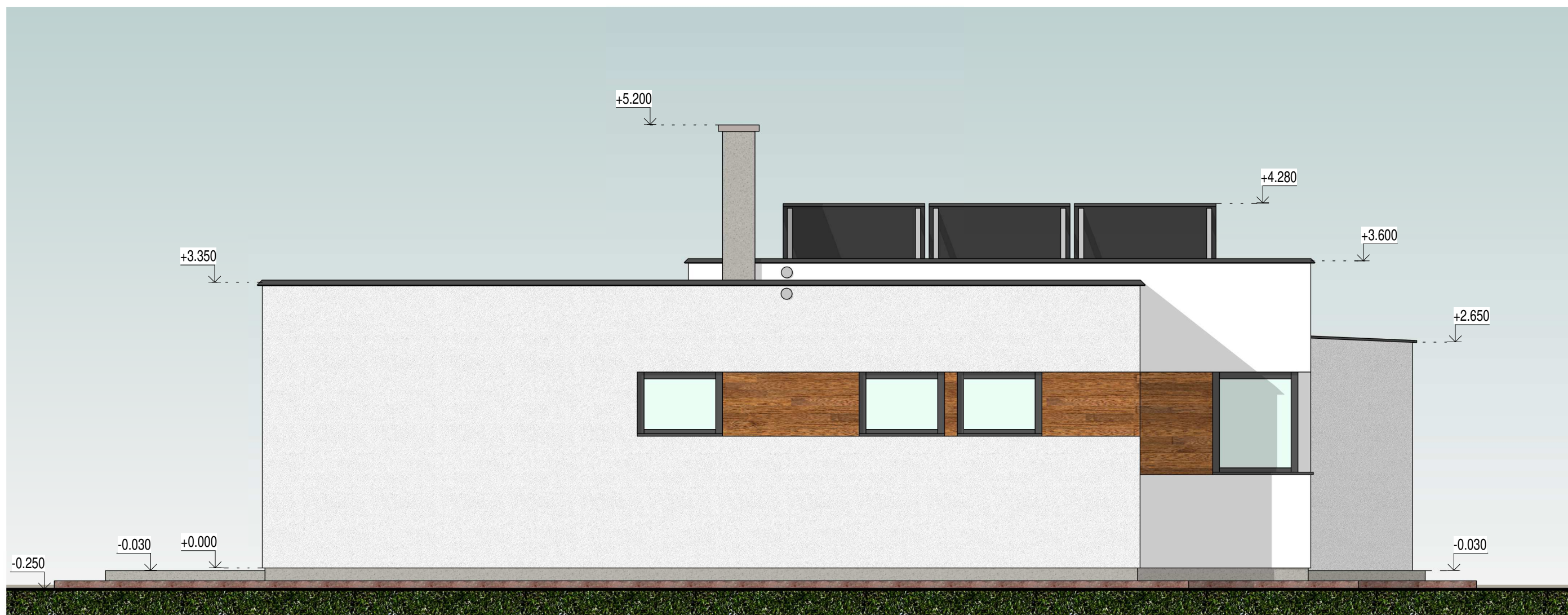
Pohľad bočný z ľava - navrhovaný stav
